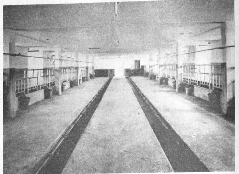
Schwenkbarer Schrägförderer, der ein Verteilen des Stallmistes über die ganze Fläche der Dunglege ermöglicht.
