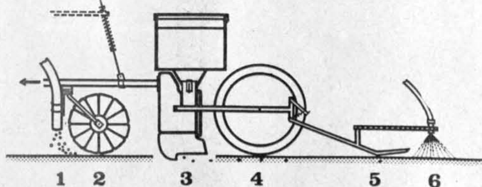
Die Anordnung der einzelnen Teile der „Multi-Culta“-Maschine für Einzelkornsaat und zum Ausdünnen: 1. Reihendüngung, 2. Krümelwalze, 3. Einzelkorn-Säapparat, 4. Druckrolle, 5. Zustrreicher, 6. Bandspritzeneinrichtung.
