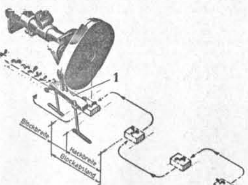
Der Schwingmesser-Ausdünnner mit einstellbarer Blockbreite läßt jeweils einen Block mit den darin gewachsenen Pflanzen stehen.
