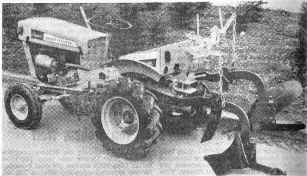
Bild oben: Kleinschlepper mit luftgekühltem 8-PS-Vergasermotor. Bild unten: Anbau-Wechselflug am Kleinschlepper „Elf“, hier mit Handaushebung; auf Wunsch wird eine hydraulische Hubvorrichtung geliefert. Schleppertypen, die auch bei der Frankfurter DLG-Ausstellung 1966 gezeigt wurden. Die DLG-Schau 1968 findet in München statt.
