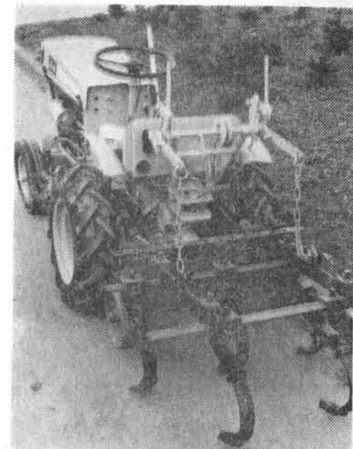
8-PS-Kleinschlepper mit fünfzinkigem Kultivator und Handhebel zum Ausheben. Zur Tiefenbegrenzung dienen zwei Stützräder.
