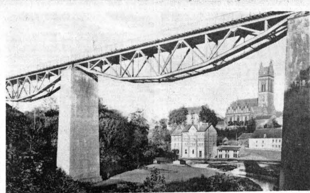
Die Eisenbahnbrücke über das Walschtal
