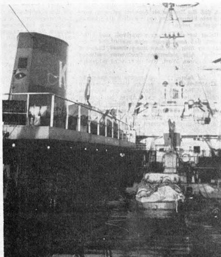
Ungewohnt mutet auf den ersten Blick die Konstruktion des Heckfängers „Jochen Homann“ an: Wie bei einem Flugzeugträger ist der Schornstein auf eine Bordseite verschoben. Damit ist mitschiffs mehr Platz für den Fisch.
