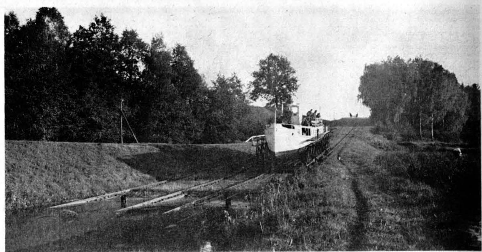
Nur in Ostpreußen und Amerika zu finden: Schiefe Ebenen zur Überwindung des Höhenunterschiedes zwischen Seen. Hier bei Schönfeld im ostpreußischen Oberland. Foto: Schultz
