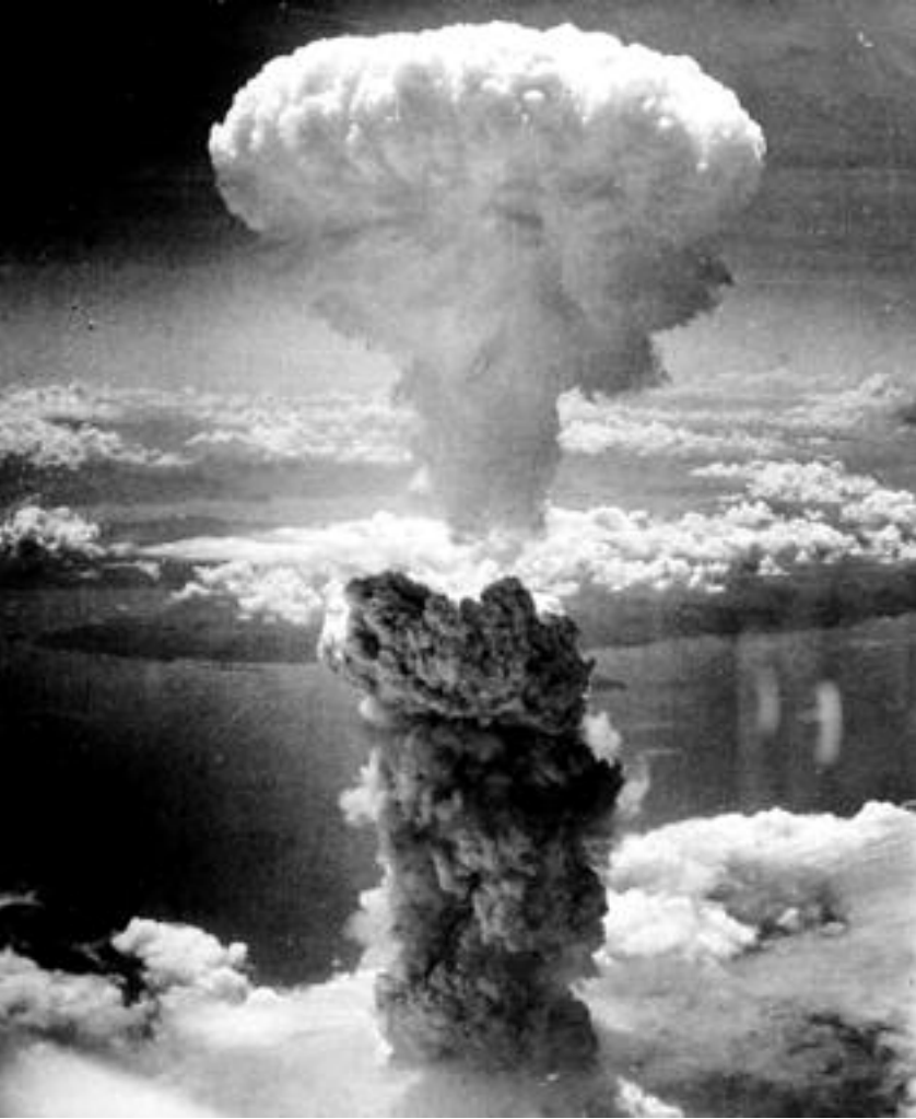
Folge des Manhattan-Projekts: Atompilz nach einer Sprengung
