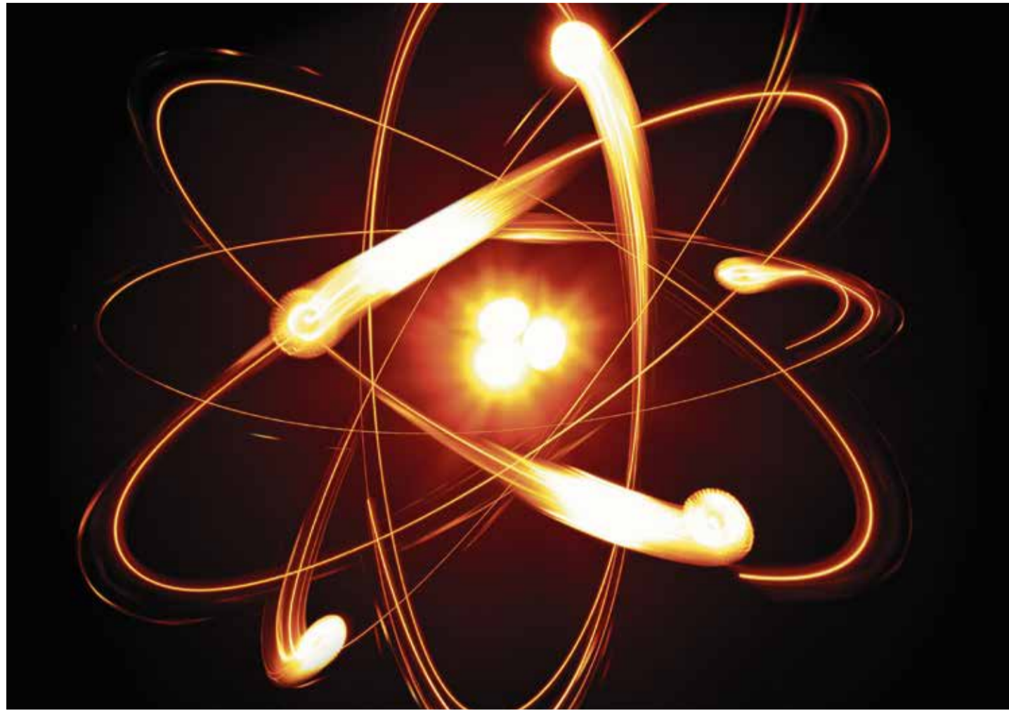
Anschauliche Illustration des Vorgangs einer Kernfusion
